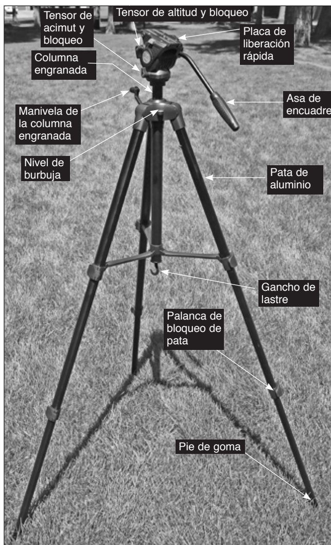
Figura 1. Trípode de campo Tritech II con las patas extendidas
