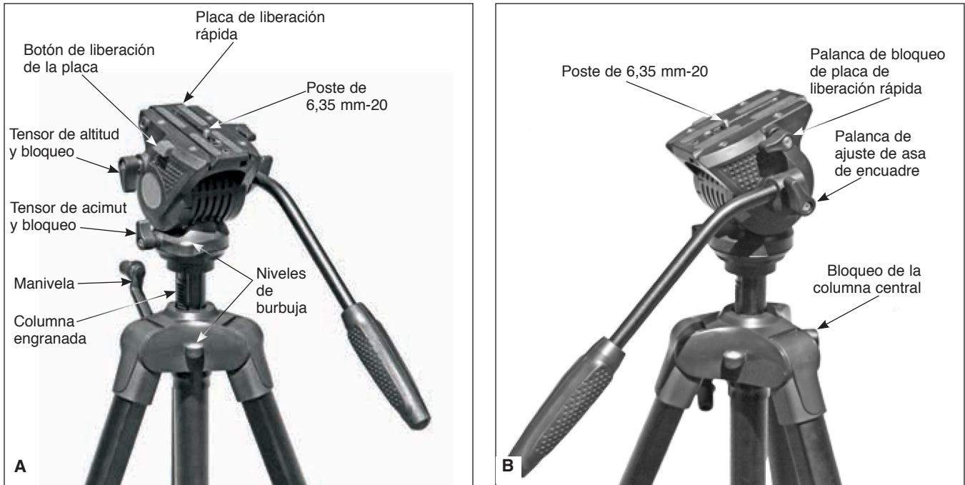
Figura 2. (A) Cabezal plano del Tritech II, lado izquierdo y (B) lado derecho.
