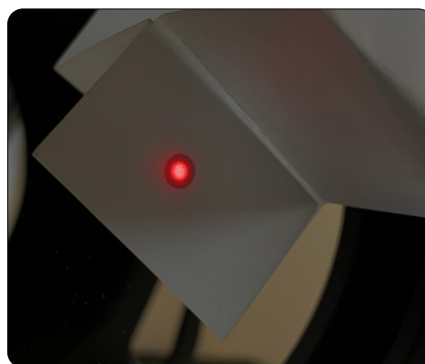
Zug- (groß) und Druckschrauben (oberes Bild); Laserpunkt und Mittenmarkierung vor und nach dem Einstellen des Okularauszugflansches.
