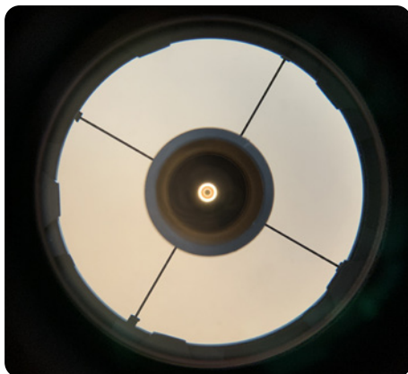
RC-Teleskop mit korrekt eingestelltem Sekundärspiegel, aber dejustiertem Hauptspiegel; TSCOLLIT-G2 auf Fangspiegelspinne scharfgestellt.
