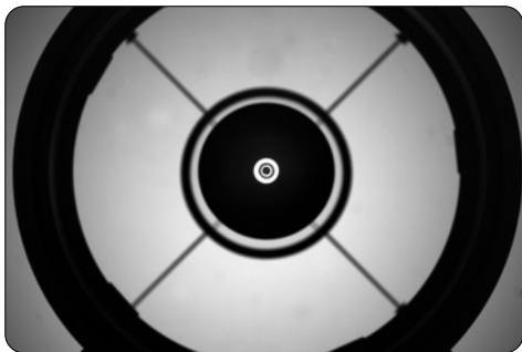
RC-Teleskop mit korrekt eingestelltem Sekundärspiegel, aber leicht dejustiertem Hauptspiegel; TSCOLLIT-G2 auf Mittenmarkierung scharfgestellt.
