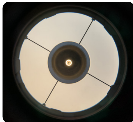
Justiertes RC-Teleskop, TSCOLLIT-G2 auf Fangspiegelspinne scharfgestellt.
