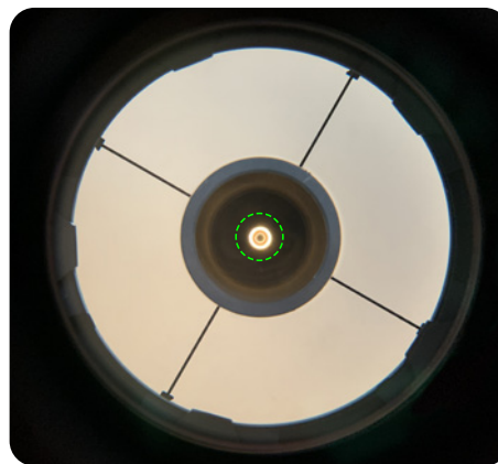
Korrekt justiertes RC-Teleskop
