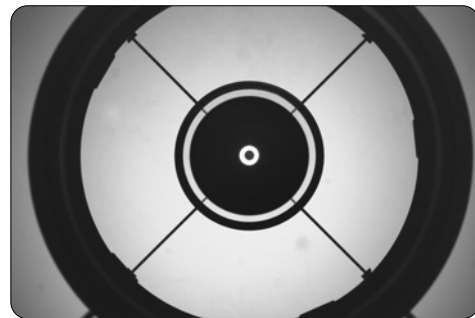
Justiertes RC-Teleskop, TSCOLLIT-G2 auf Fangspiegelhalter scharfgestellt.
